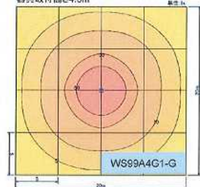
水平面参考照度分布図 器具取付高さ4.5m
